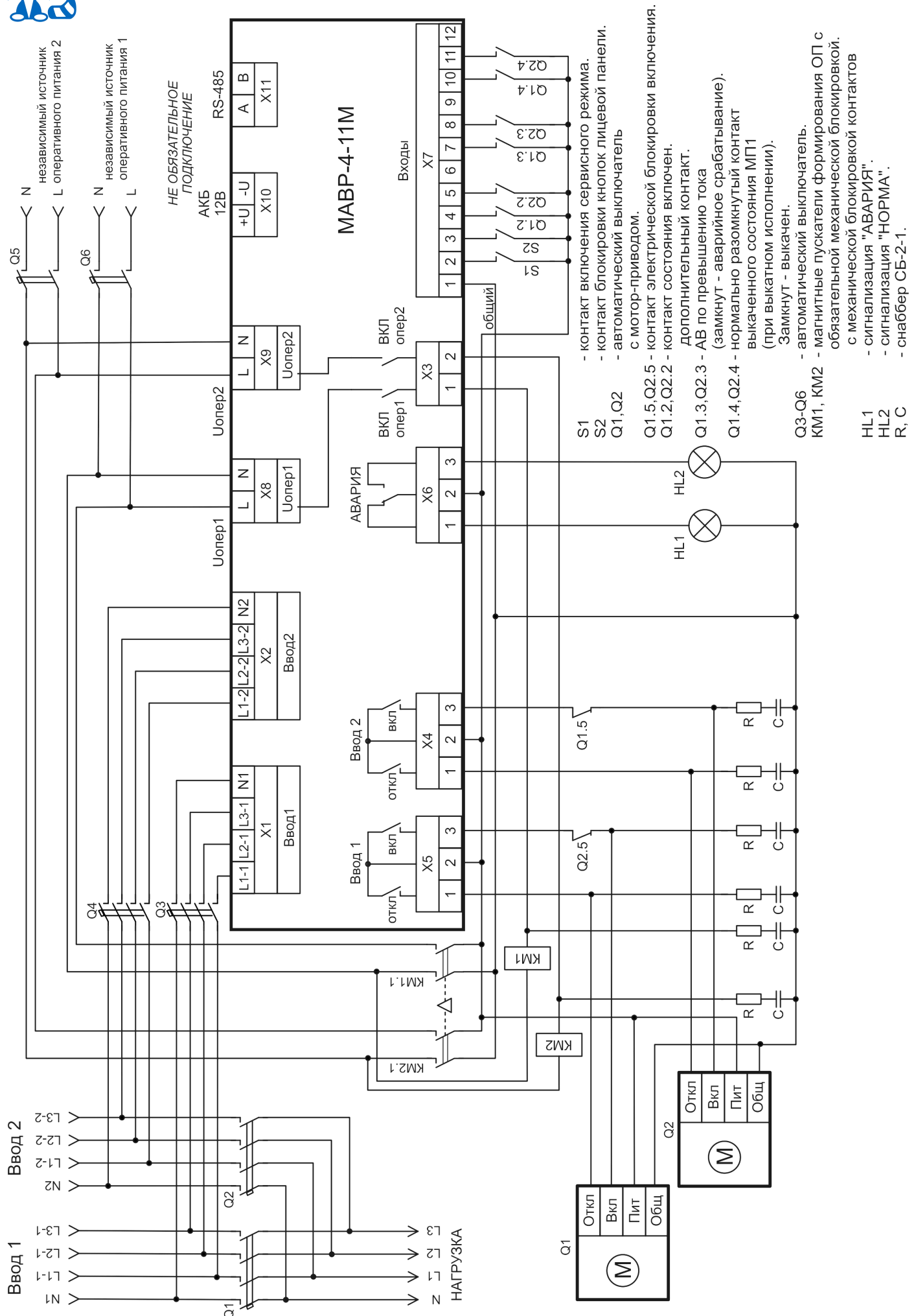
Рис.9 Схема АВР на автоматических выключателях
