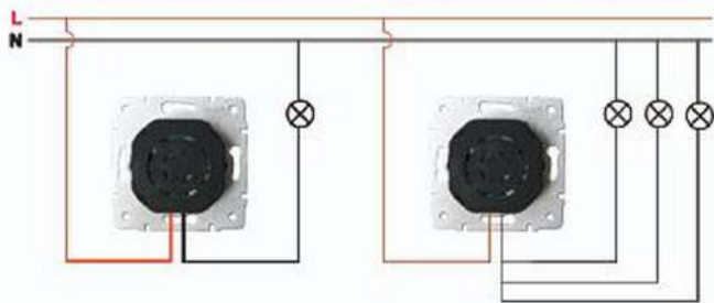
Схема подсоединения / Connection Diagram
